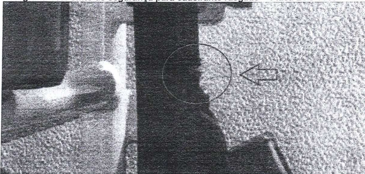
Fotografia 119. Cinto de segurança para cadeirante rasgado - Placa EVU 1669
