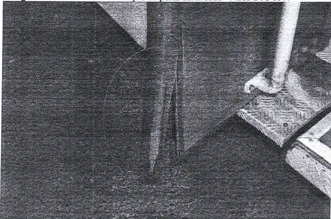
Fotografia 107. Borracha de vedação da porta danificada - Placa DVS 8511
