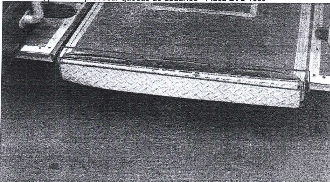
Fotografia 118. Plataforma elevatória com cantoneira/revestimento de degrau danificada, podendo provocar quedas de usuários - Placa EVU 1669
