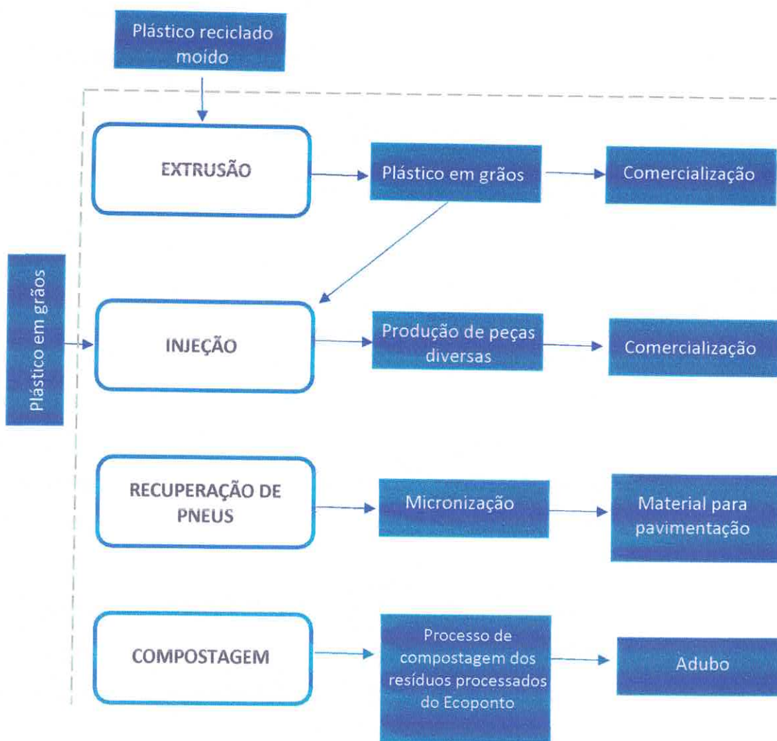
Figura 1 – Fluxograma simplificado do processo produtivo da STL Plastic
