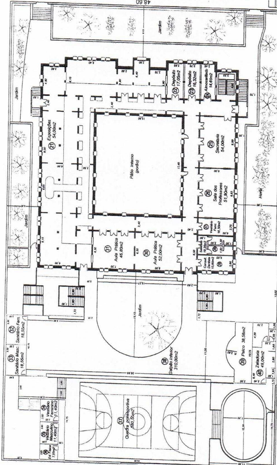
Planta - Pavimento Inferior - esc. 1:100
